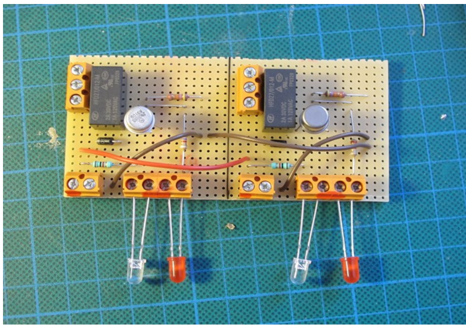
Illustration 58: Réalisation carte électronique pour passerelle de détection [GSR_23]
