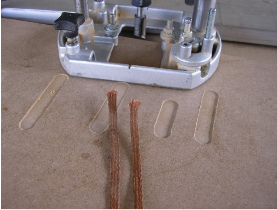
Figure 1: Essais de profondeur de rainure d'encastrement de tresse
