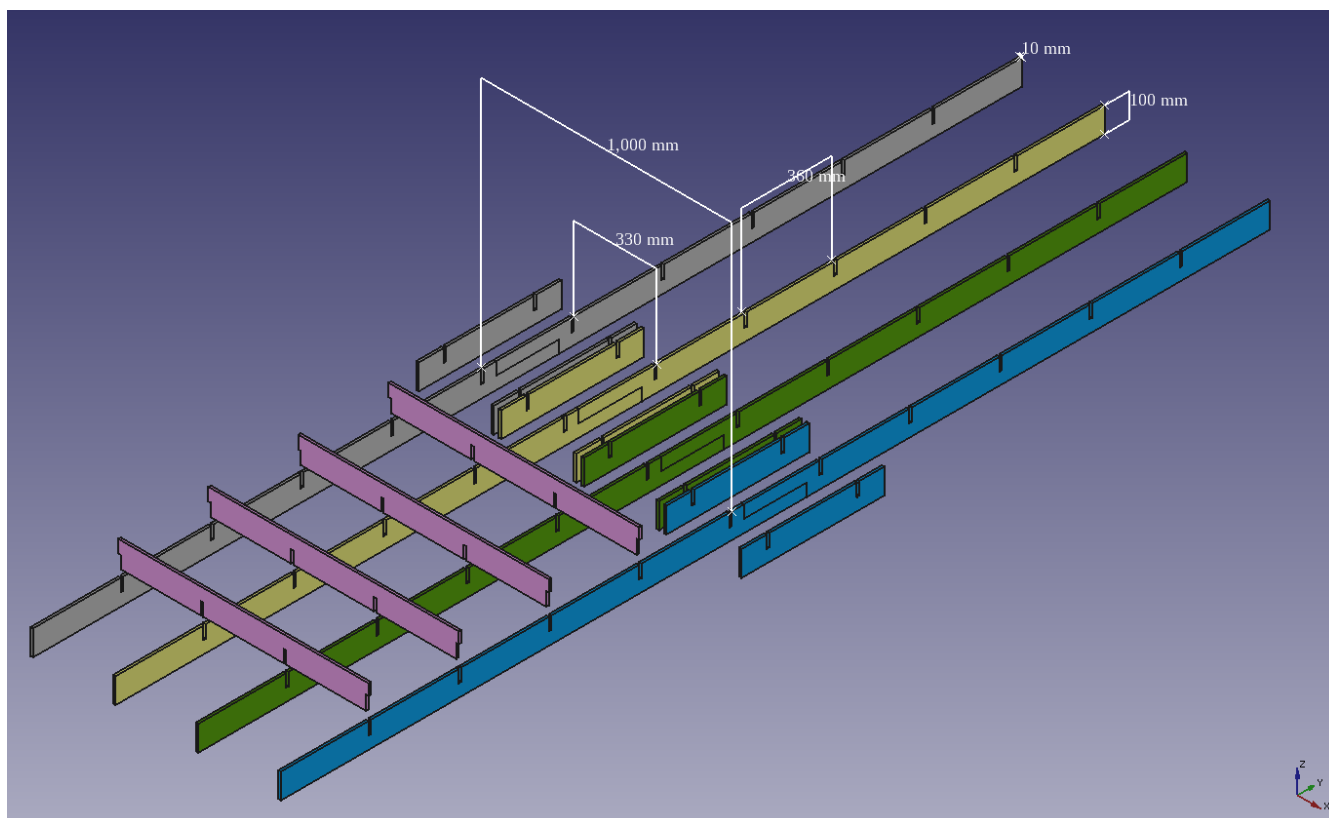
Illustration 32: Structure treillis coupe mi-bois pour ossature suspendue
