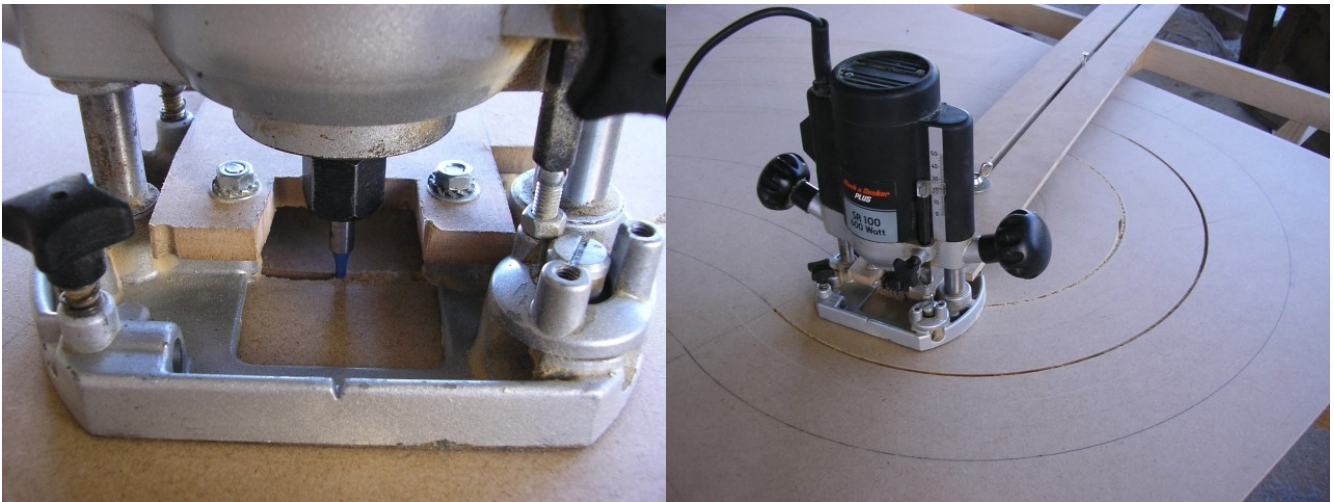
Illustration 4: Compas pour défonceuse [GSR_05]
