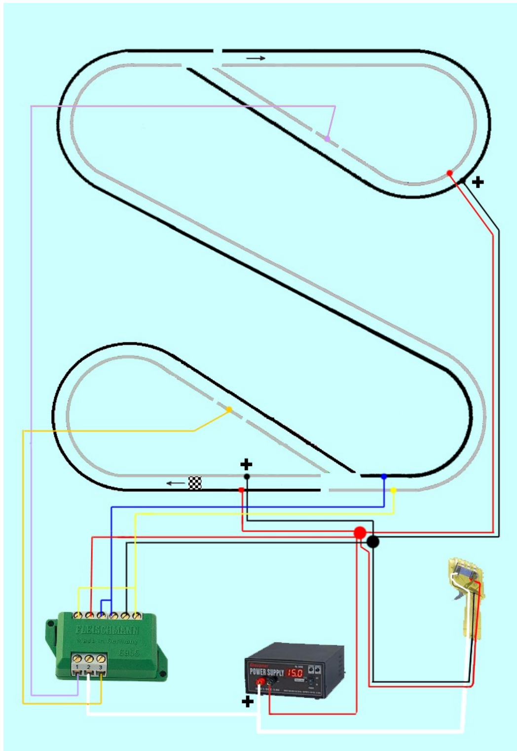
Illustration 64: Boucle de retournement par relais inverseur double (Ph. Point)
