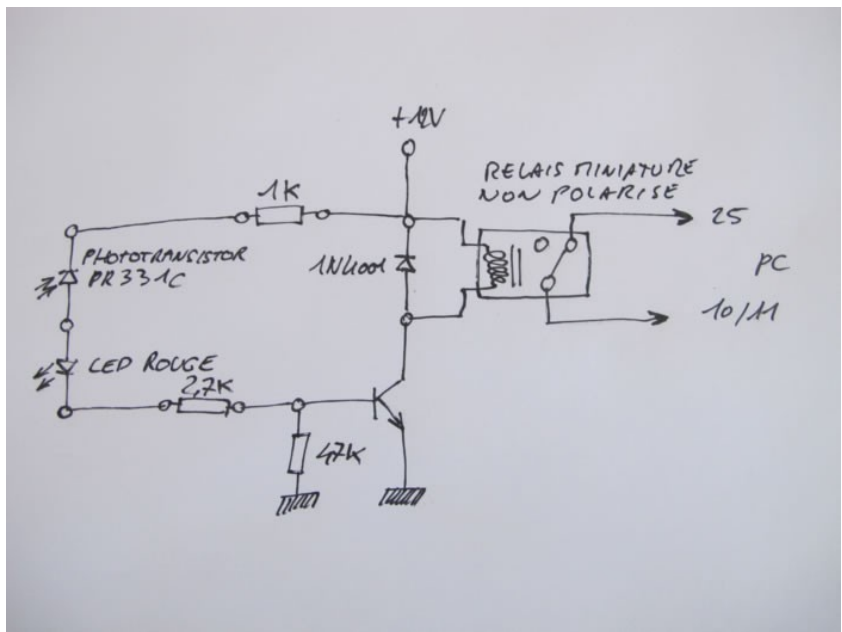
Illustration 57: Schéma électrique pour passerelle de détection [GSR_23]
