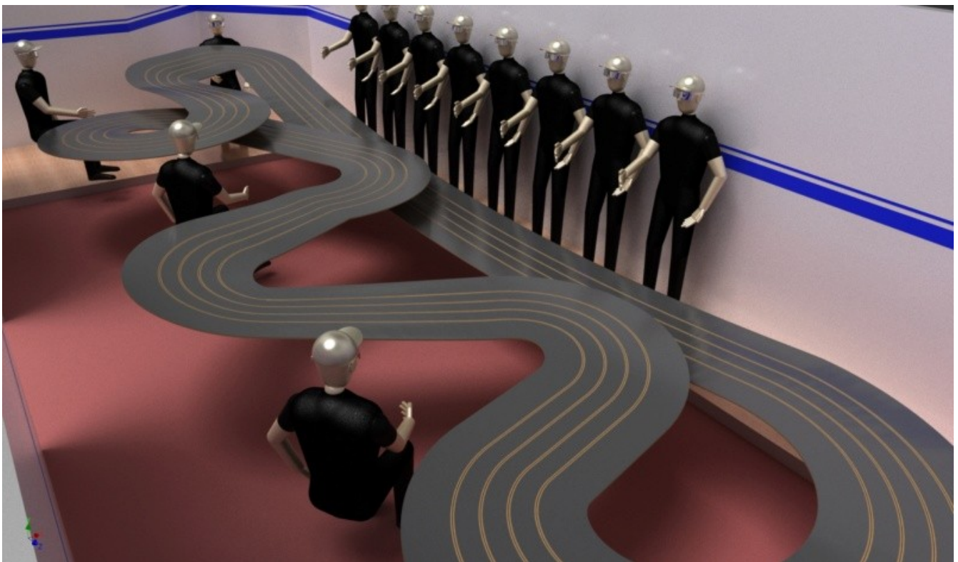
Illustration 15: Conception CAO 3D piste bois Cirso32 (vue dessus) [GSR_15]
