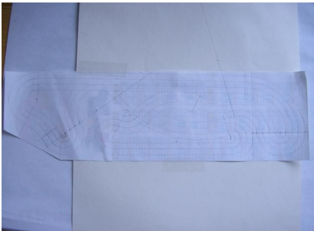
Illustration 12: Exemple de dessin de piste à l'échelle 1/10 ième [GSR_05]
