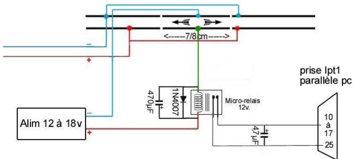
Illustration 61: Schéma de détection par dead-strip selon Ph. Point
