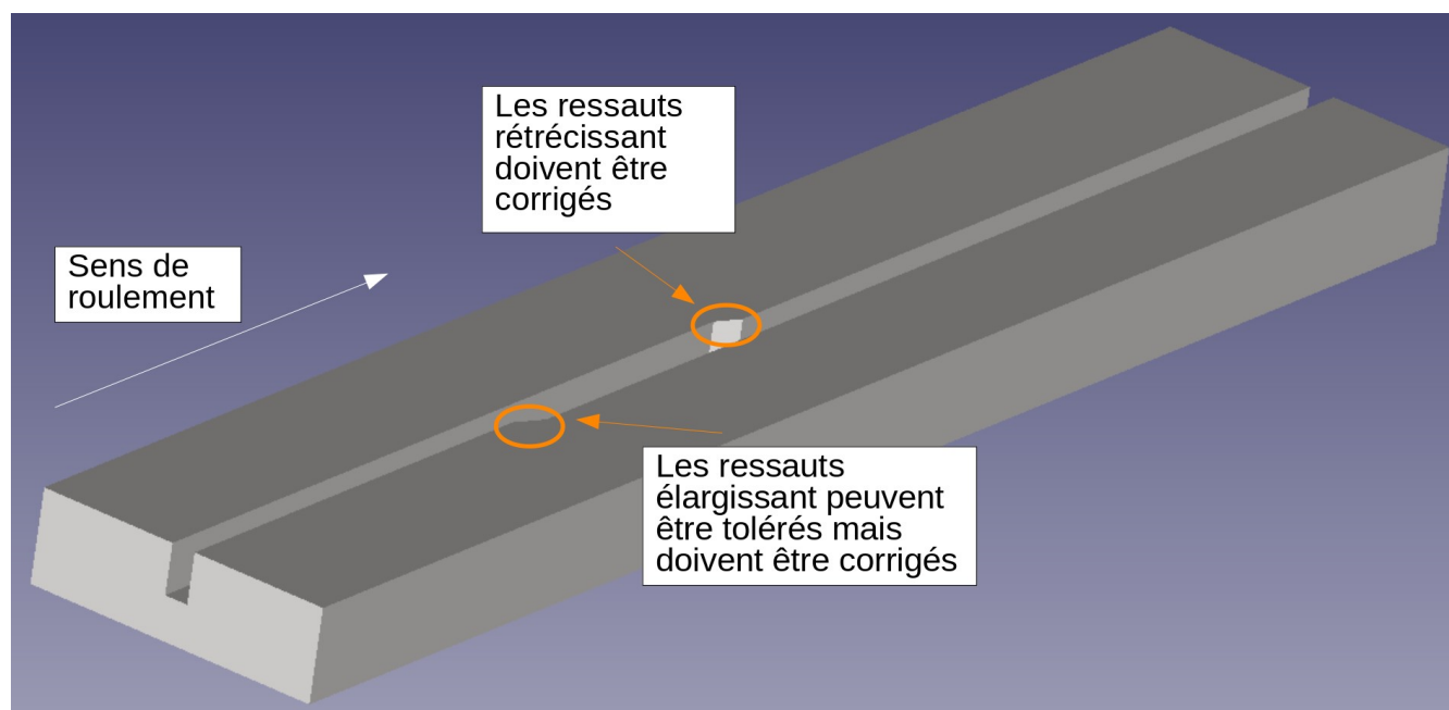
Illustration 43: Correction des rétrécissements, élargissements dans la fente
