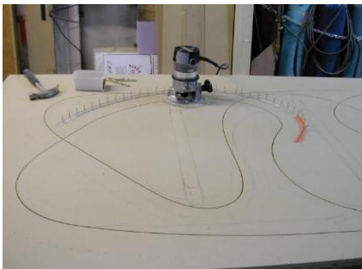
Illustration 1: Le guide de défonçage "routing kit" de Luf [GSR_02]
