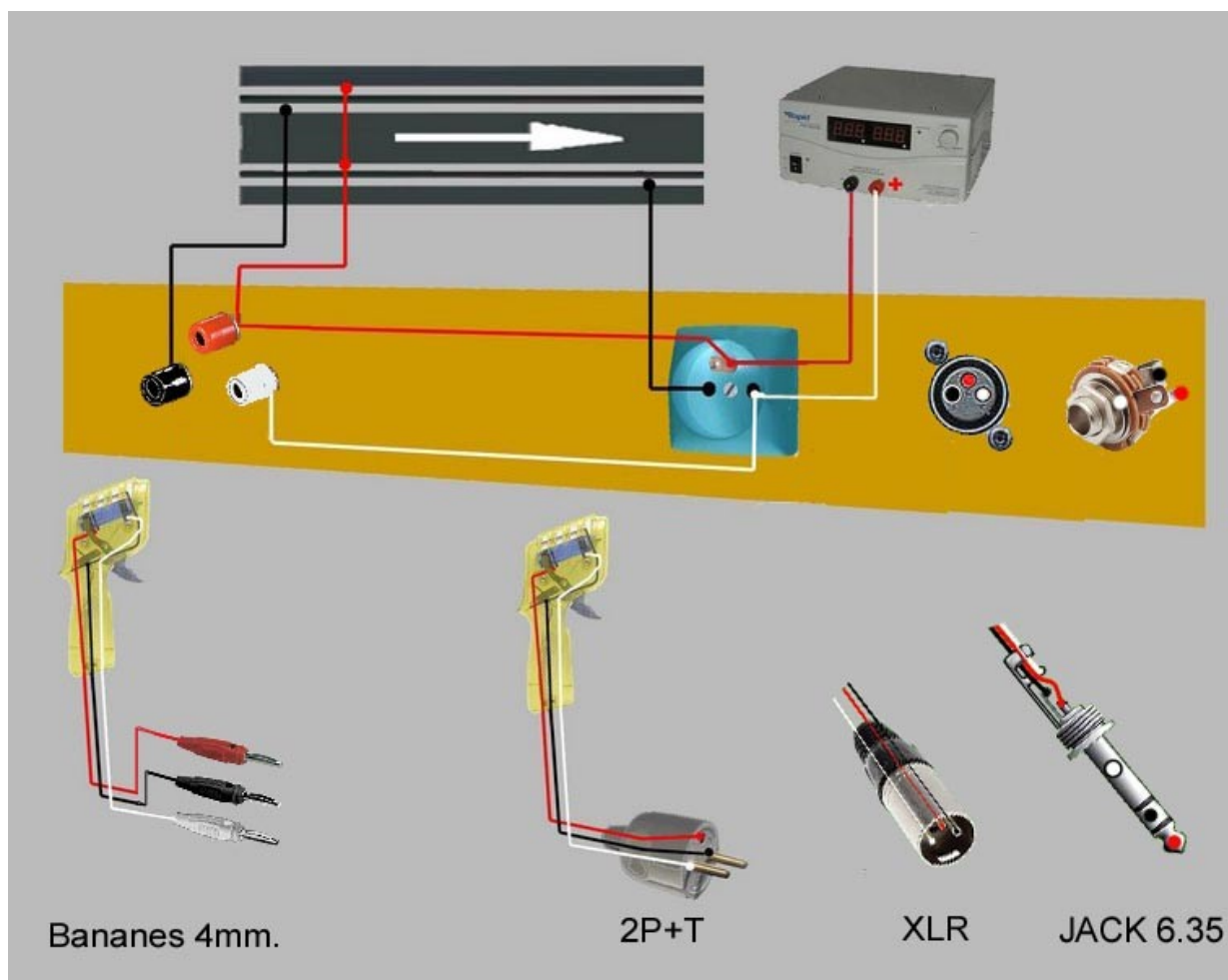
Illustration 55: Branchement pour différents types de prises bananes, xlr, etc. par Ph. Point.
