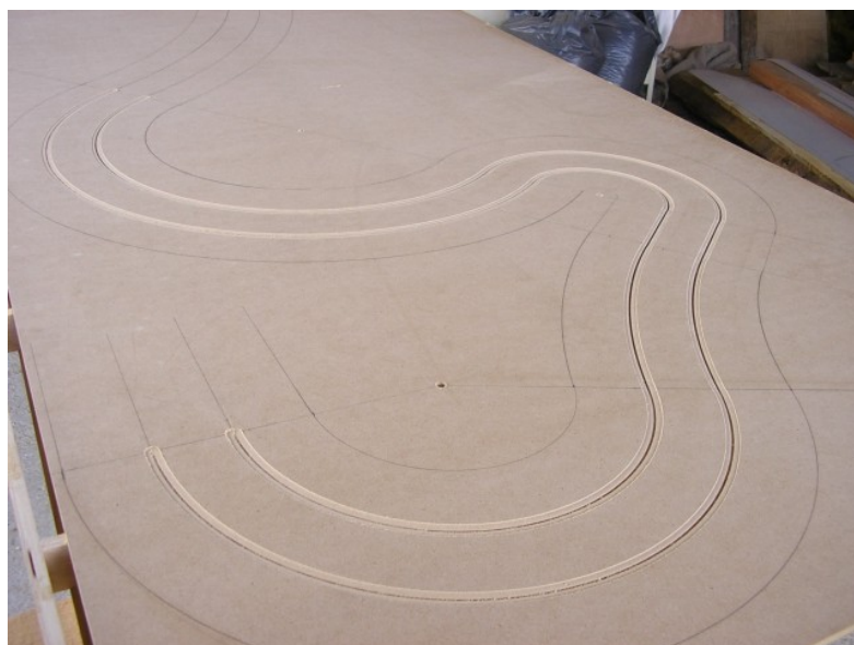
Illustration 22: Tracé prêt à être défoncé et résultat du défonçage
