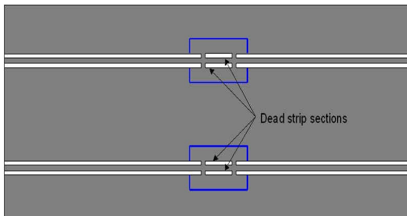
Illustration 60: Zone de détection par coupure (dead strip)
