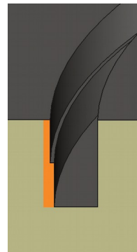
Illustration 39: Supprimer les ressauts dans la fente
