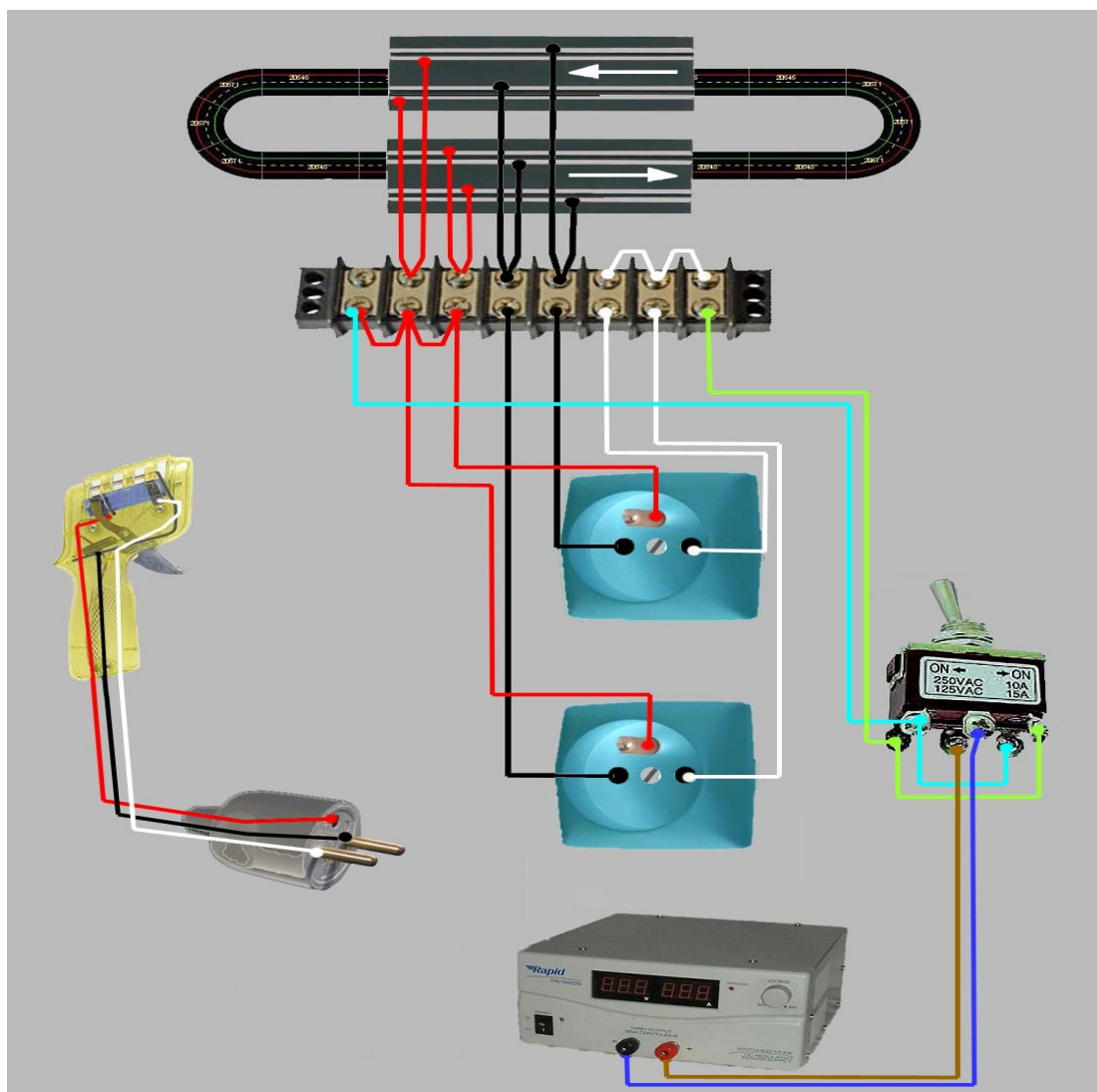
Illustration 54: Branchement poignée piste avec inverseur de sens [GSR_18]
