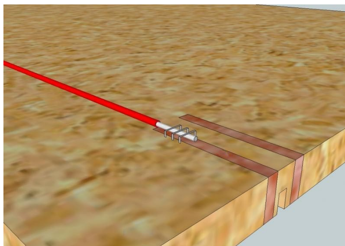
Illustration 53: Raccordement bande de cuivre
