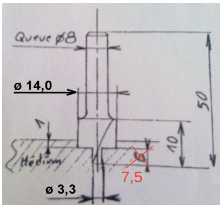
Illustration 8: Schéma de commande d'une double fraise sur mesure [GSR_06]
