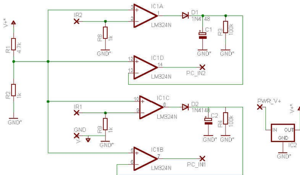
Illustration 62: Carte électronique de détection par dead-strip [GSR_24]
