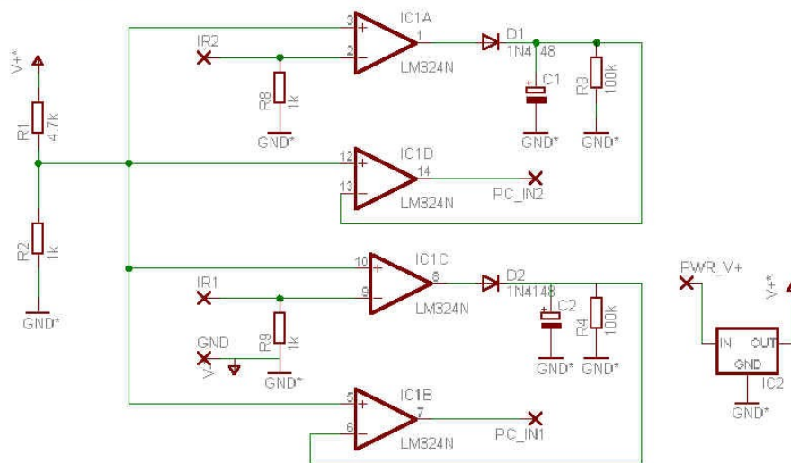
Illustration 59: Carte électronique de détection par passerelle [GSR_24]
