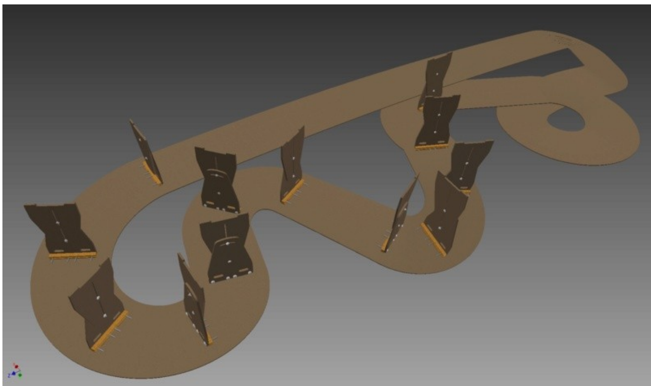
Illustration 16: Conception CAO 3D piste bois Cirso32 (vue dessous) [GSR_15]
