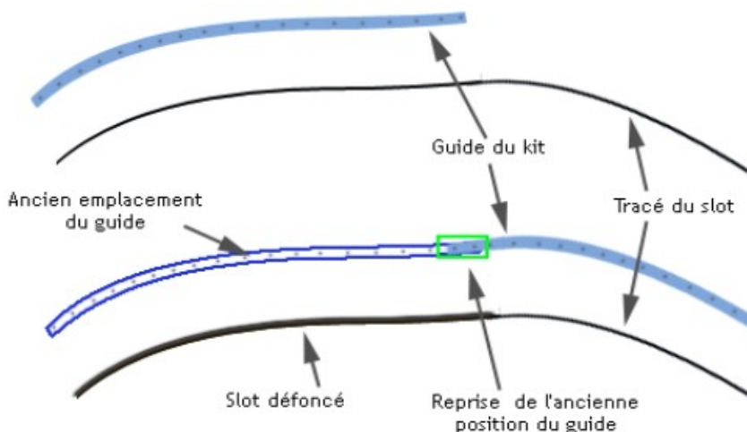
Illustration 38: Utilisation du guide Lexan
